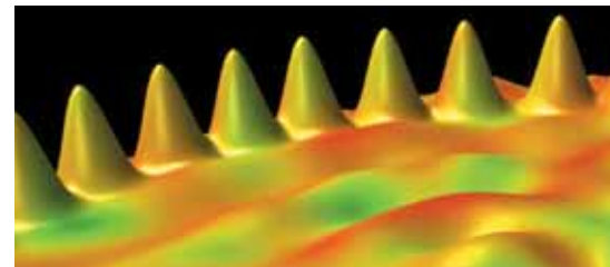
Kunstvoll arrangierte Atome auf einer Metalloberfläche: Die Atome erscheinen als Kegel, die ein Oval bilden, 5.000 mal kleiner als der Durchmesser eines menschlichen Haars. (Bild: IBM Almaden Research Center, USA)
